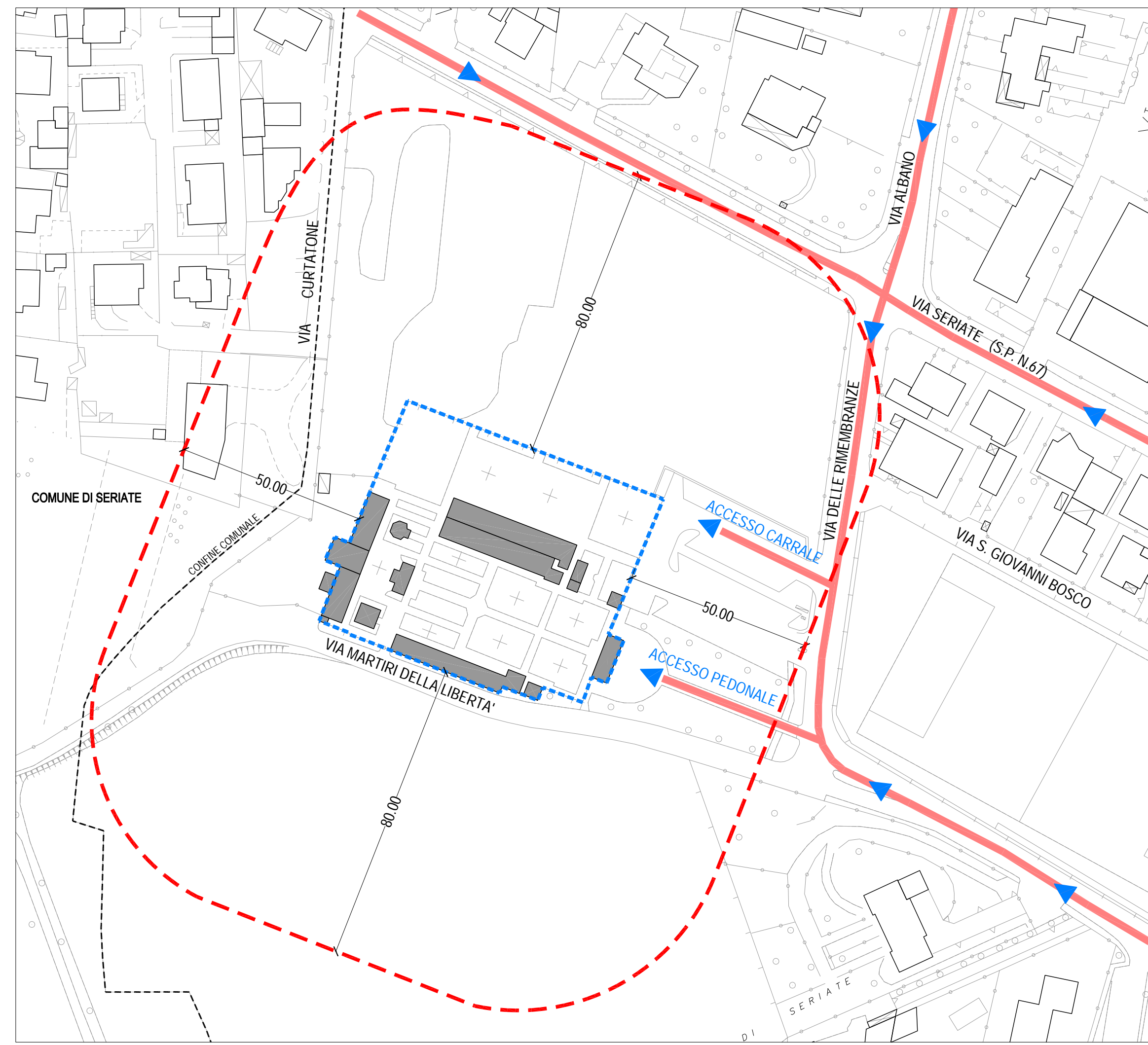
PLANIMETRIA GENERALE scala 1:1.000
